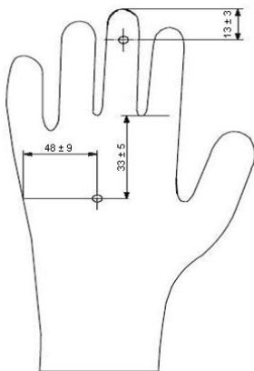
Figura A.2 - Pontos de medição para espessura da luva
